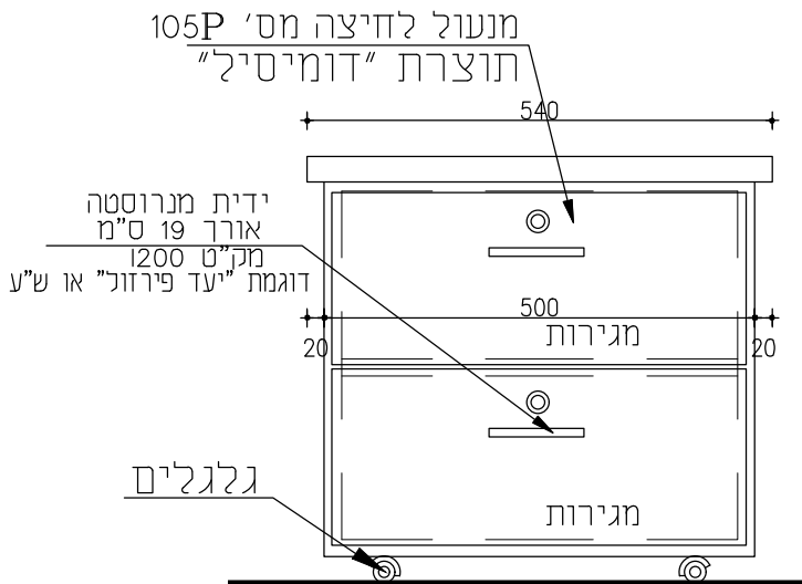
מבט 1 קנ"מ 1:10
