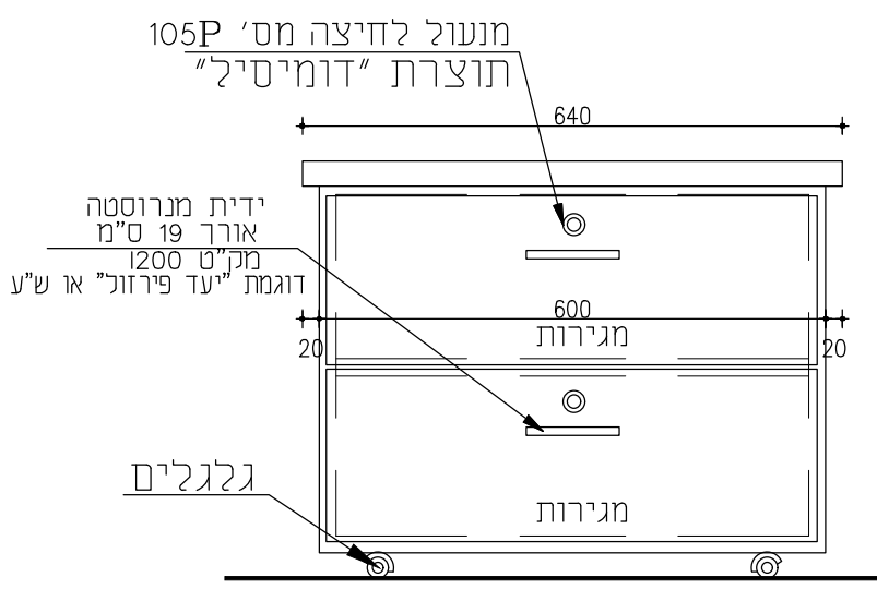
מבט 1 קני"מ 1:10
